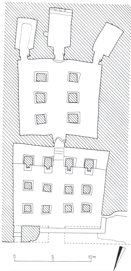
Abb. 6: Grundriss des Tempels von Derr (nach Hein, Rames- sidische Bautätigkeit, Taf. 9).
