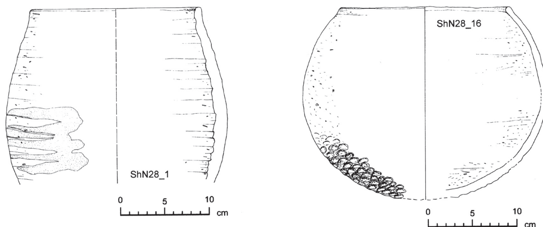
Abb. 3 Beispiele für Keramik aus Kuppelgräbern (Zeichnung: J. Budka)
