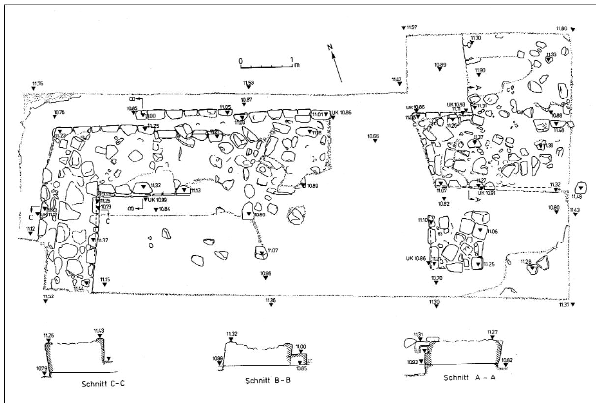
Abb. 2: Schnitte 601.N1 und 601.24: Planumszeichnung der Reste des Nordtores von Hof 601 (Feldzeichnung: C. Hof, Umzeichnung: I. Säuberlich).
