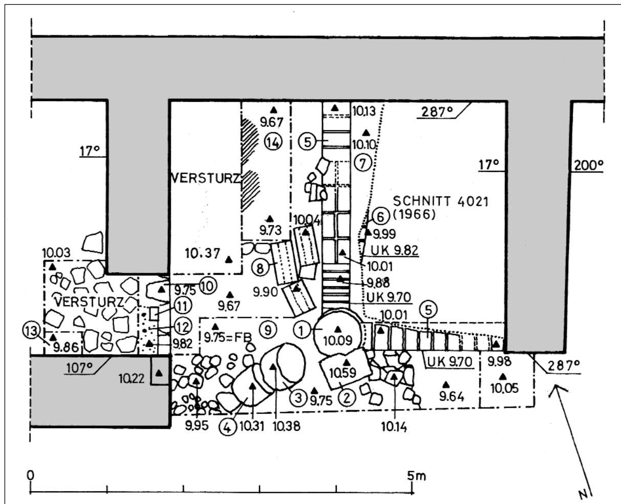
Abb. 7: Schnitt 402.2, Planum nach Abschluß der Freileigungsarbeiten.
