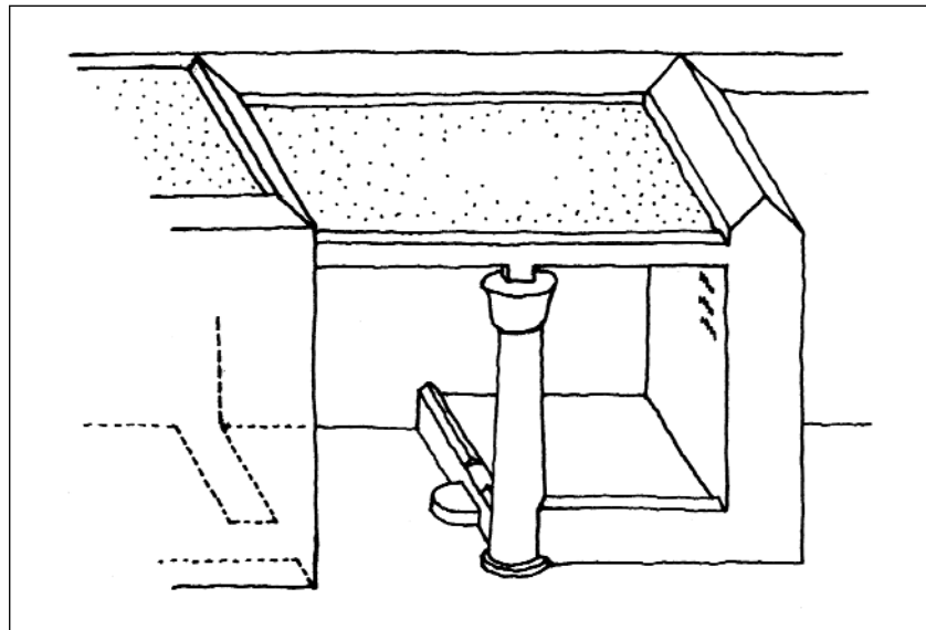
Abb. 12: Zeichnerische Rekonstruktion des Raumes 402 (Vorschlag). Die Lage der Graffiti an Wand 402/406 ist angegeben.
