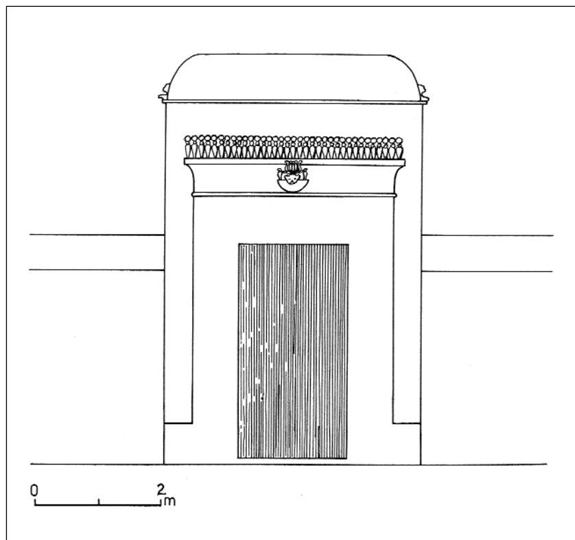
Abb. 14: Rekonstruktionsvorschlag für die Ansicht des Haupttores 305/E des Großen Anlage. In der Hohlkehle über der Toröffnung ist das „Emblem des Apedemak“ angebracht. An den Schmalseiten des Torbaues sitzt je ein Löwenprotom über der Traufplatte in der untersten Lage des Eselsrückens (Entwurf: D. Eigner, Zeichnung: I. Säuberlich).
