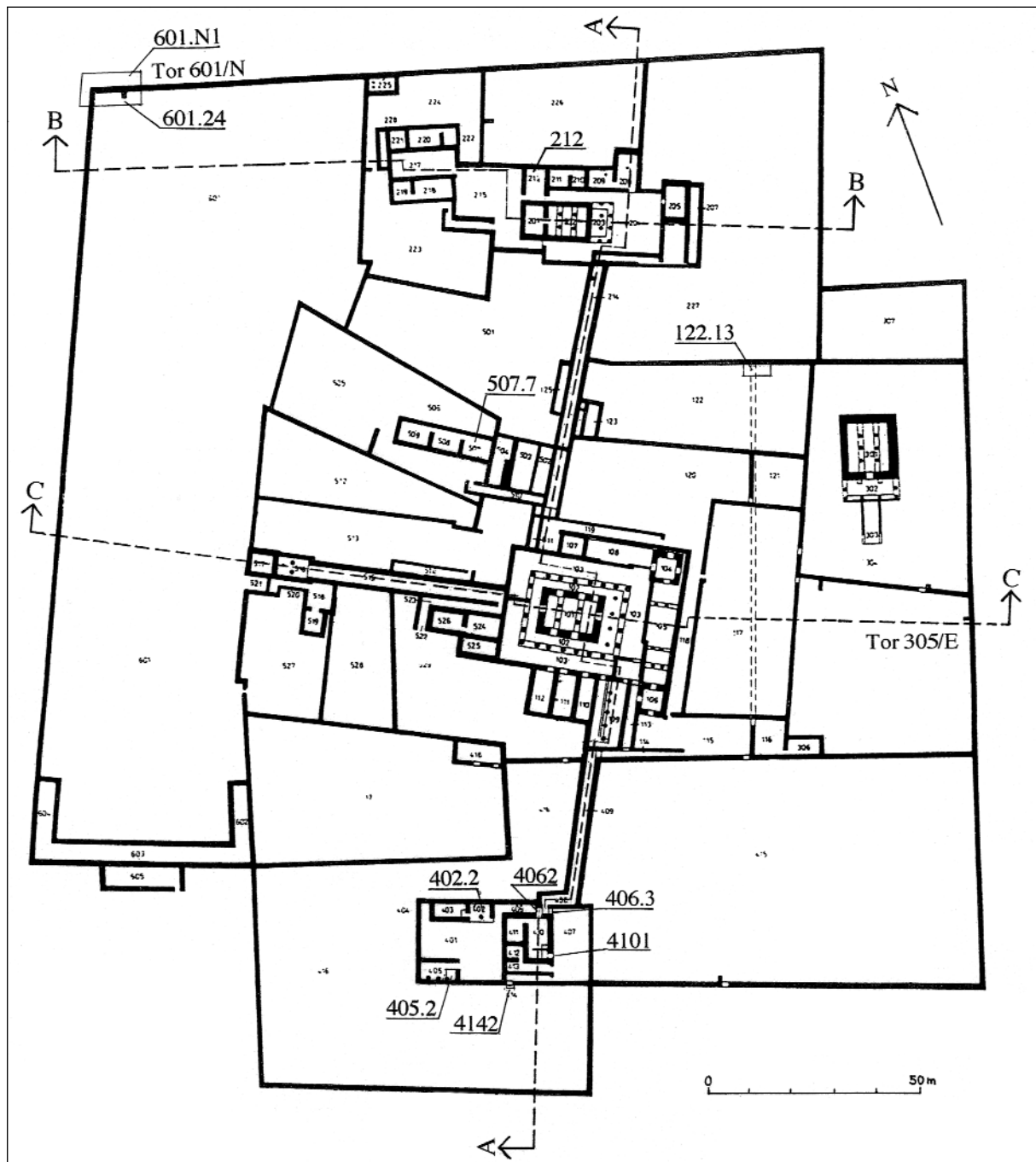
Abb. 1: Plan der Großen Anlage. Eingetragen sind Lage und Nummern der im Bericht besprochenen Schnitte und Sondagen, sowie die Lage der geplanten Schnittzeichnungen (A-A, B-B, C-C), die Lage des Säulen-Raumes 212 und des Tores 305/E.
