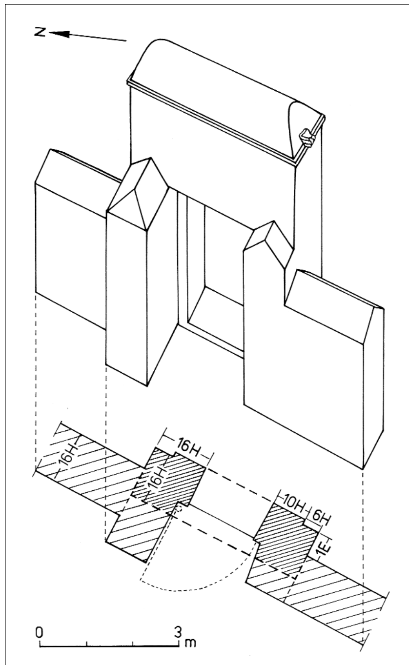
Abb. 15: Rekonstruktionsvorschlag für den Torbau 305/E, Vogelschau auf die Innenseite (Entwurf: D. Eigner, Zeichnung: I. Säuberlich).
