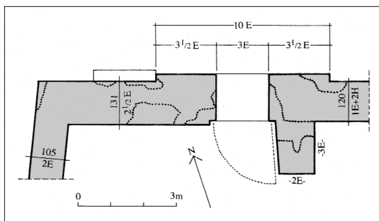
Abb. 5: Vorschlag für die Rekonstruktion des Grundrisses von Nordtor Hof 601.
