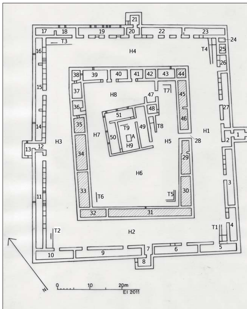
Abb. 10: Orientierungsplan. Die Räume sind im Uhrzeigersinn mit fortlaufenden Nummern versehen. H – Höfe, T – Treppen, Rampen, A – „Altar“ (Zeichnung: D. Eigner).
