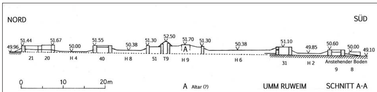
Abb. 5: Schnittzeichnung A – A zu Plan Abb. 4 (Feldaufnahme D. Eigner & Tim Karberg, Zeichnung: D. Eigner).
