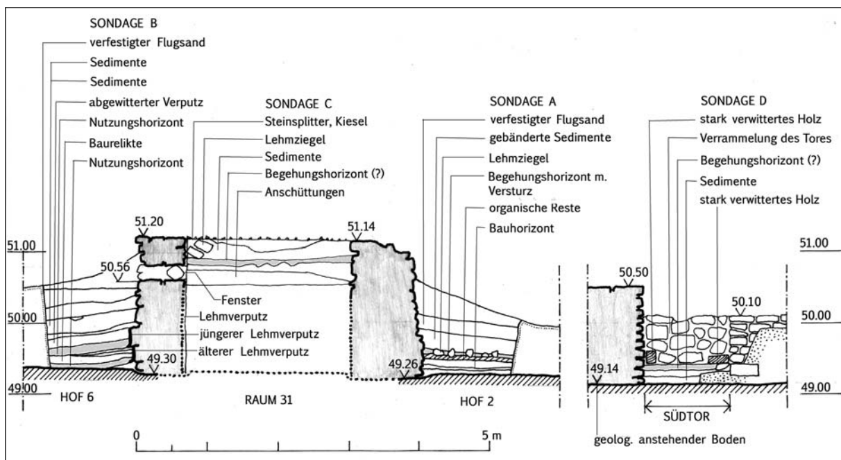
Abb. 9: Die Sondagen A, B, C und D des Testschnitts. = Südteil der Schnittzeichnung Abb. 5 inkl. des Ostprofils der Sondagen. An der Außenseite der Nordwand von Raum 31 dokumentieren zwei Verputzschichten zwei Nutzungsphasen von Hof 6 (Feldaufnahme: Tim Karberg & Laura Haupt, Umzeichnung: D. Eigner).
