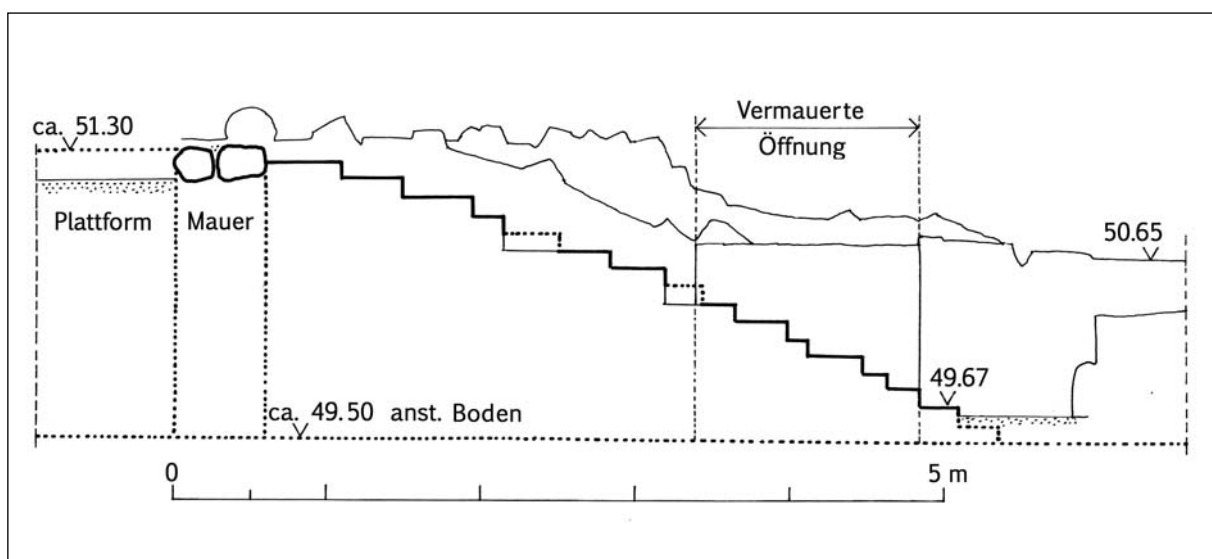
Abb. 18: Schematischer Längsschnitt durch Treppe 4. Auf 4,50 m Länge wird ein Höhenunterschied von 1,63 m überwunden. Aus diesem sehr bequemen Steigungsverhältnis ergeben sich 15 Stufen zu je 11 cm Höhe, mit 14 Auftrittsflächen von je 32 cm Breite. Die tatsächliche Ausführung ist jedoch sehr unregelmäßig und erfolgte sichtlich ohne entsprechende Planung (Zeichnung: D. Eigner).
