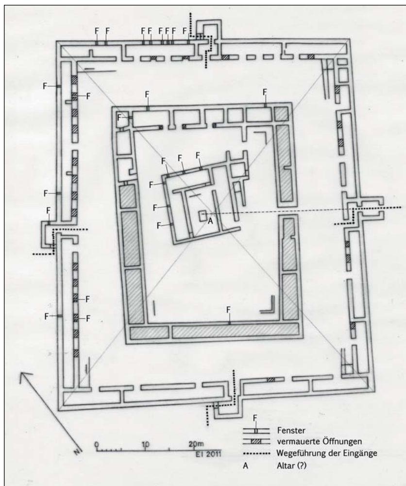
Abb. 14: Öffnungen im Mauerwerk des Baues Umm Ruweim 1: Tore, Türdurchgänge und „Fenster“. Das Haupttor der Anlage ist exakt auf den Altar (?) A ausgerichtet, welcher mit guter Genauigkeit im geometrischen Zentrum der gesamten Anlage liegt (Zeichnung: D. Eigner).
