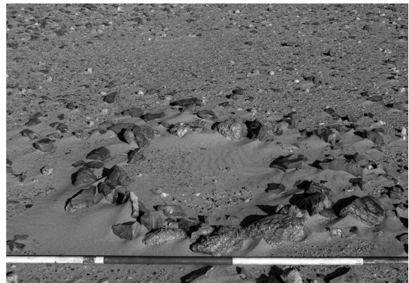
Abb. 19: Steinring 4705-1
