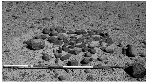
Abb. 17: Plattform 4512-6
