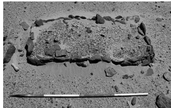
Abb. 13: Kiesbett Site 5236-1
