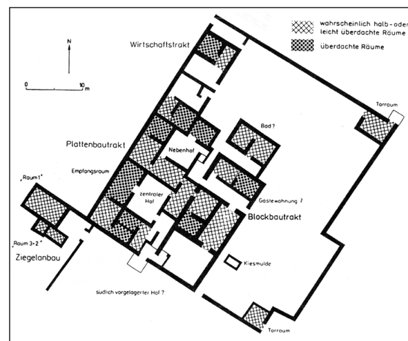
Abb. 3: Kleine Anlage, zweite Nutzungsphase (nach Fitzenreiter 1999: 187, Abb. 17/18).
