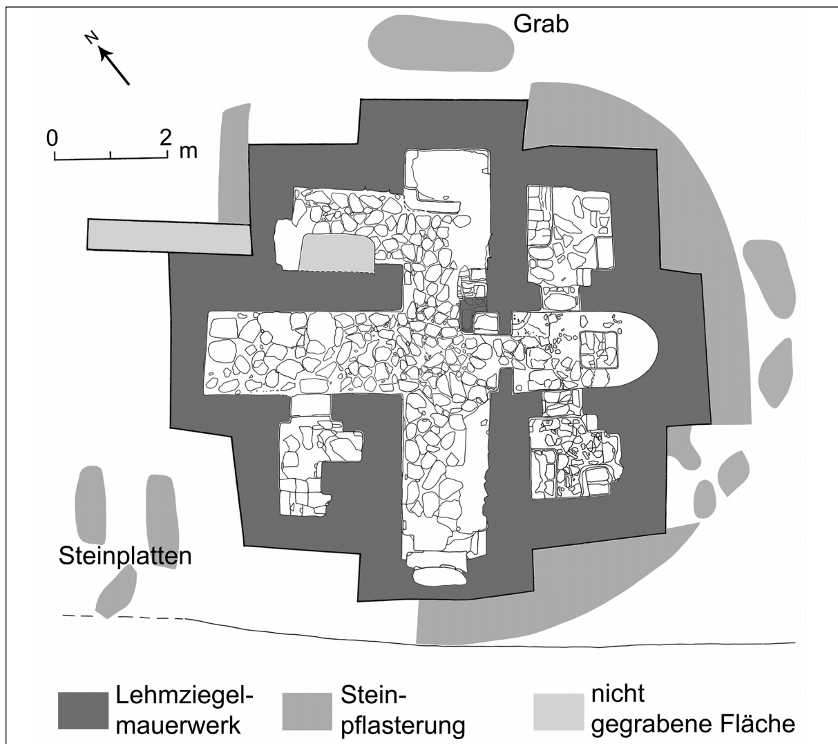
Abb. 14: Überblicksplan der Kirche US022 (Zeichnung: D. Billig / M. Lange / C. Näser; Illustration: I. Säuferlich).
