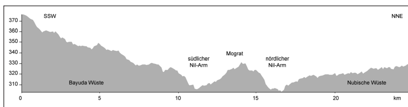
Abb. 2: Im digitalen Geländemodell lassen sich entlang des Geländeprofiles die unterschiedlichen Gefälle zum Niltal sowie die Asymmetrie der Insel erkennen (Daten: NASA 2006).
