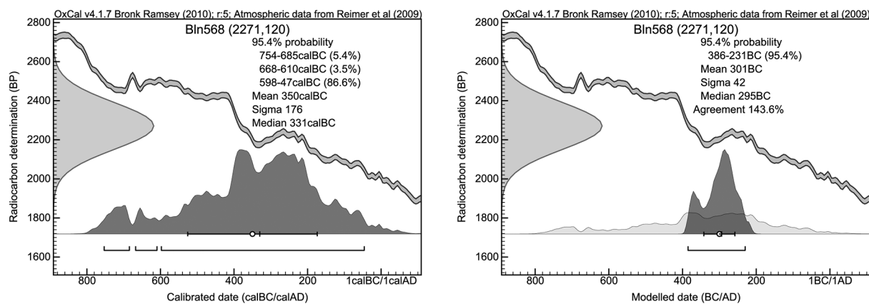
Abb. 7 und 8: Vergleich der Kalibrierungsdiagramme des unmodellierten (links; vgl. Abb. 1) und des modellierten (Modell 2, vgl. Abb. 10) ^{14}\text{C} -Datums der Probe Bln 568 (Gründungsdeposit unter der Rampenmauer 207/227). Dargestellt sind jeweils die konventionelle (BP) und die kalibrierte (cal BC) Wahrscheinlichkeitsverteilung sowie der Verlauf der Kalibrierungskurve. Im Diagramm rechts ist die modellierte Wahrscheinlichkeitsverteilung (über der x-Achse) mit der unmodellierten Verteilung (hellere Fläche) hinterlegt. Die Klammern unterhalb geben jeweils die Spanne(n) der 95,4%-Verteilung an.
