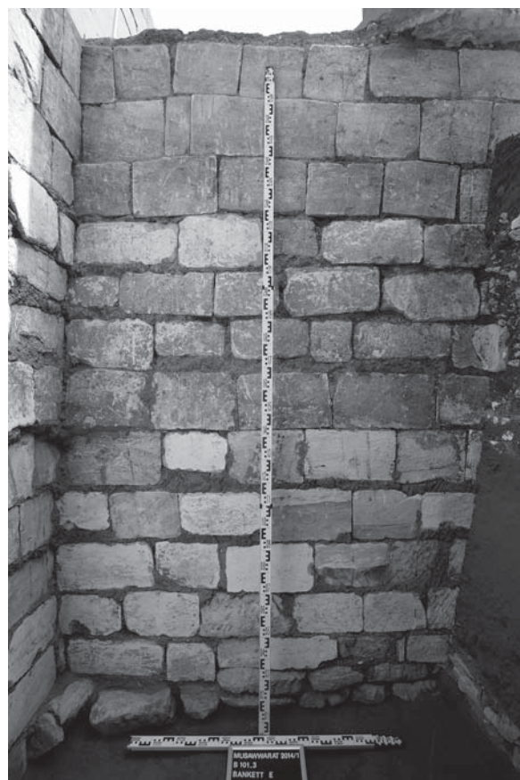
Abb. 4: Das westliche Säulenbankett an der Ostseite von Schnitt 101.3. Darunter die ein bis zwei überbauten (Fundament-)Lagen des Tempels der Bauperiode 3 (Foto: Scheibner).
