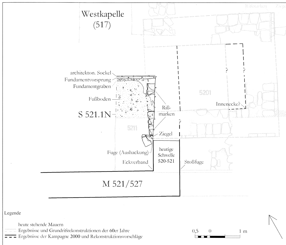
Plan I. Grundlagen: P-IA/51 (Zeichnung Stark), P-IA/111=Plan VII aus Hintze 1971 (Zeichnung Stark 1968/69), P-IA/533 (Zeichnung Mucha 2000).
